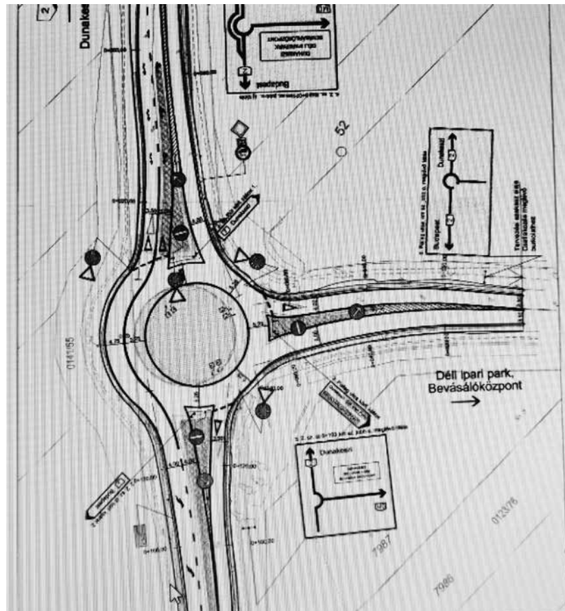
A város déli határában kétsávosra bővül a főút és a két körforgalmi csomópont dunai oldala
